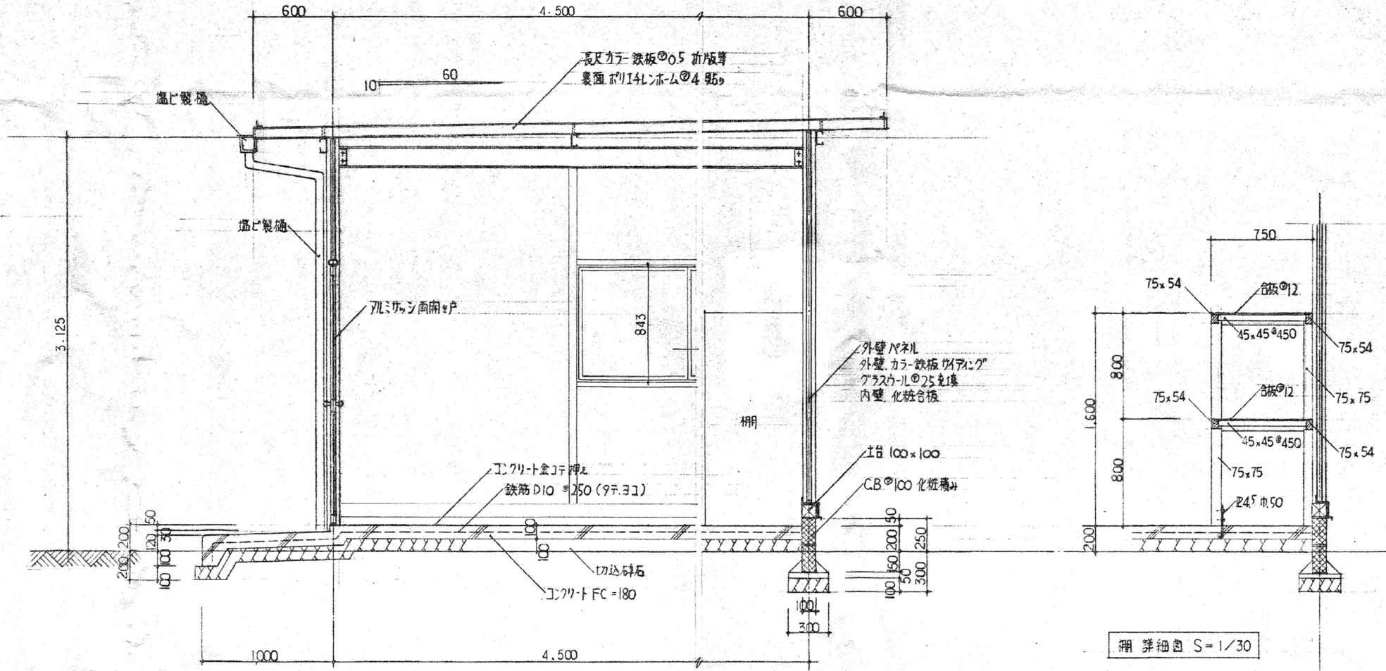
断面図 S=1/30
