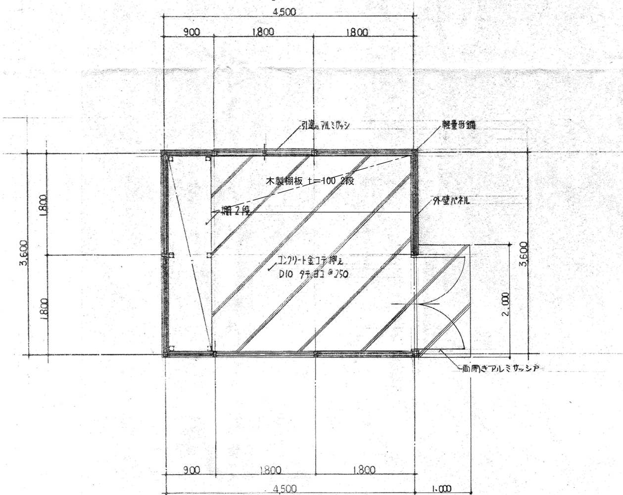
平面図 S=1/50
