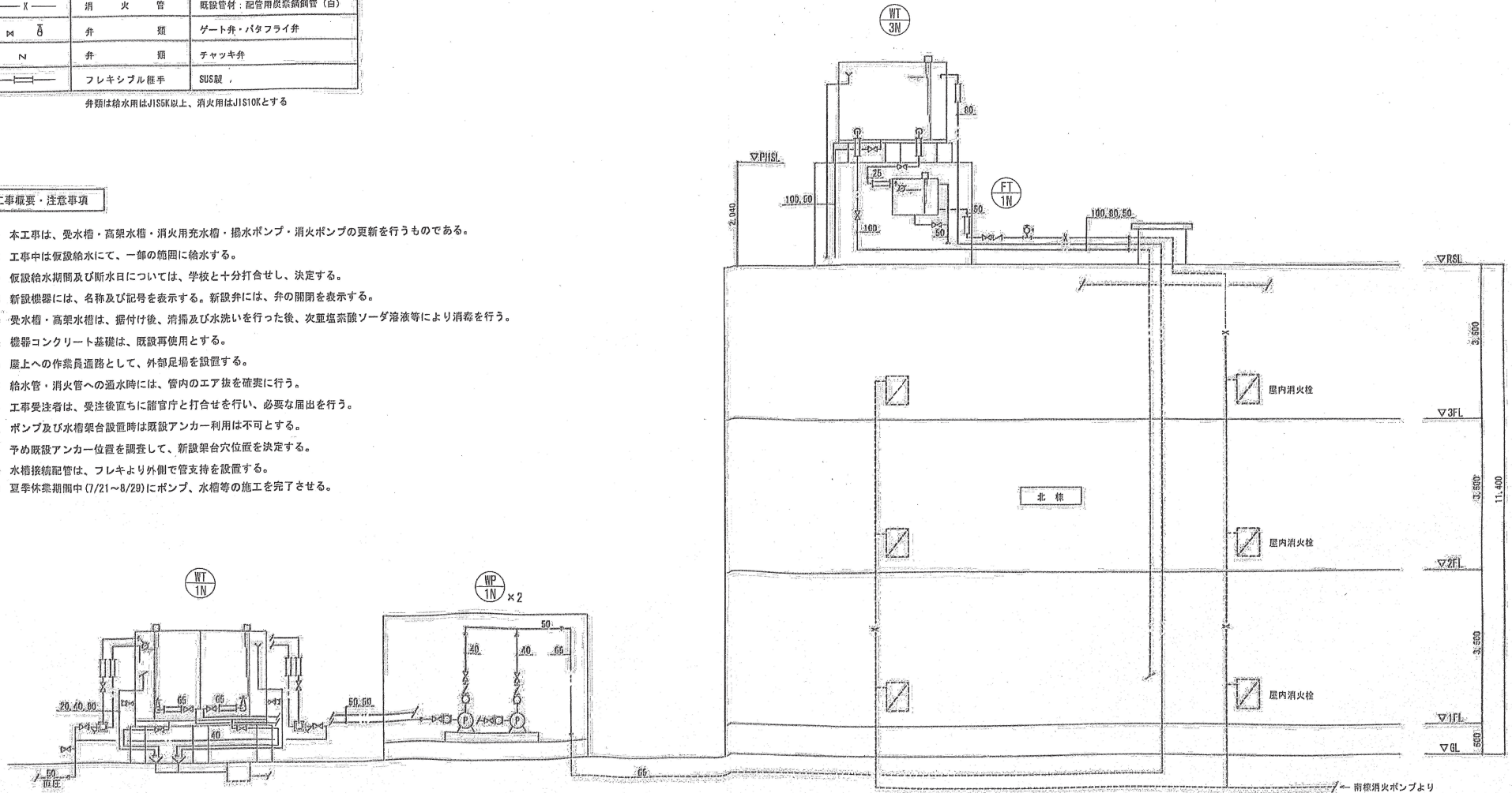
系統図 (北棟)
