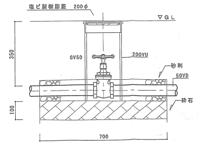
仕切弁廻り詳細図 1/10
