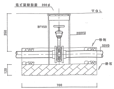
バタフライ弁廻り詳細図 1/10
