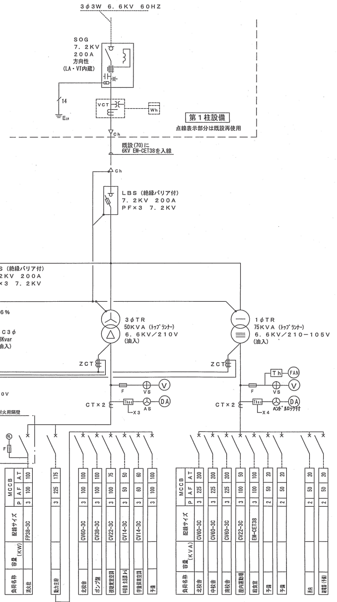
受電キュービクル(改修後) 単線結線図
