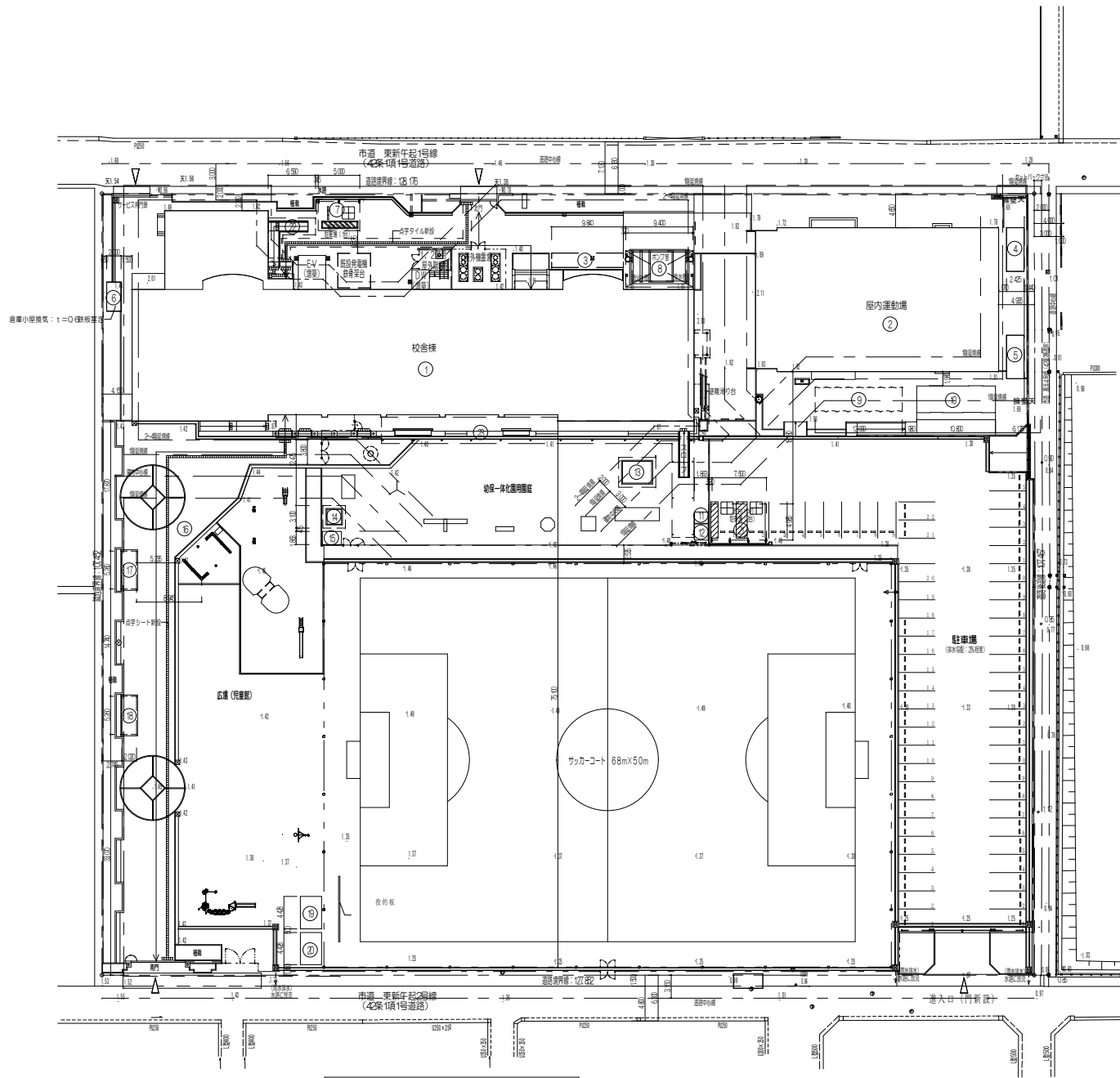
配置図 S=1/600 (A3)
