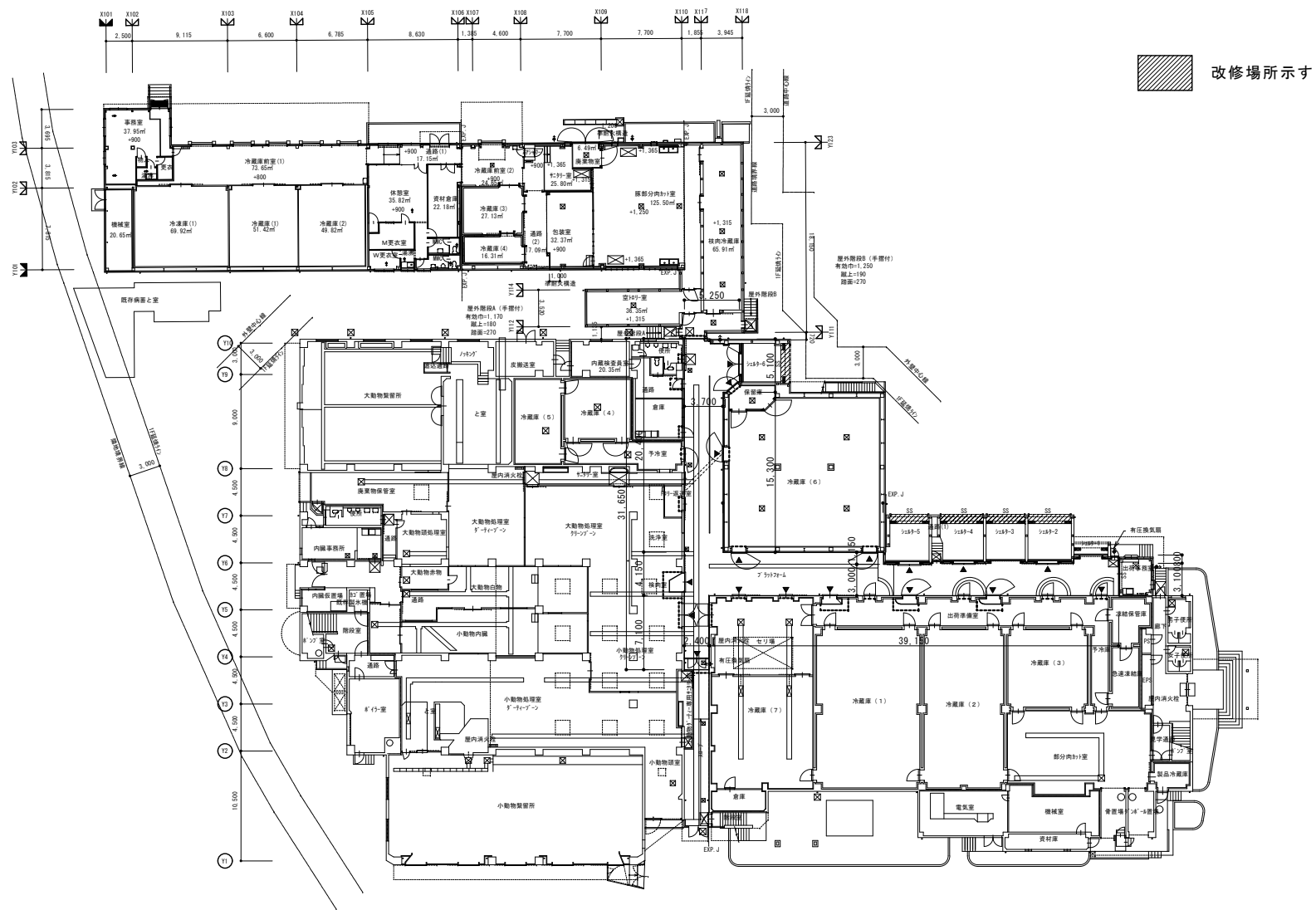
1階平面図
