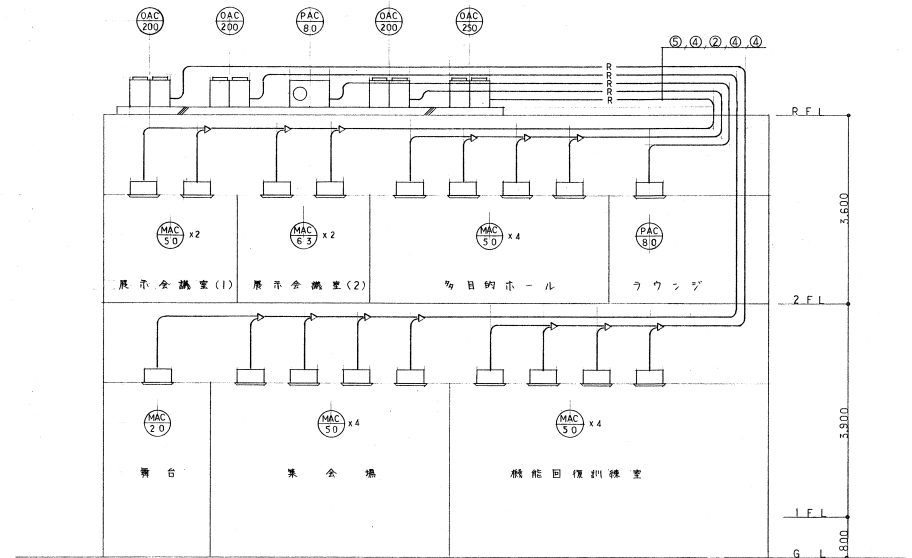
空調配管系統図 NO SCALE
