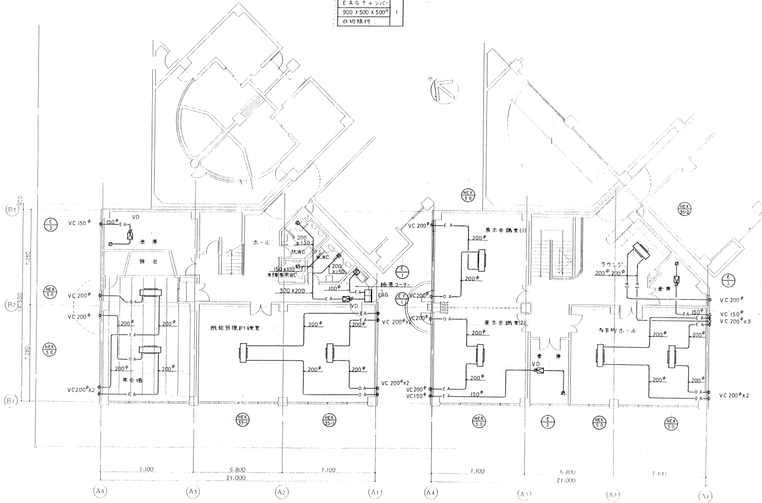
1階ダクト平面図 S: 1/100
