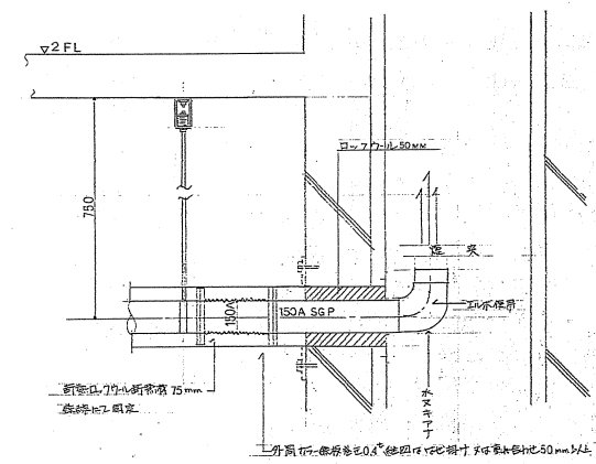
排水管 取組寸法詳細図 1/10
