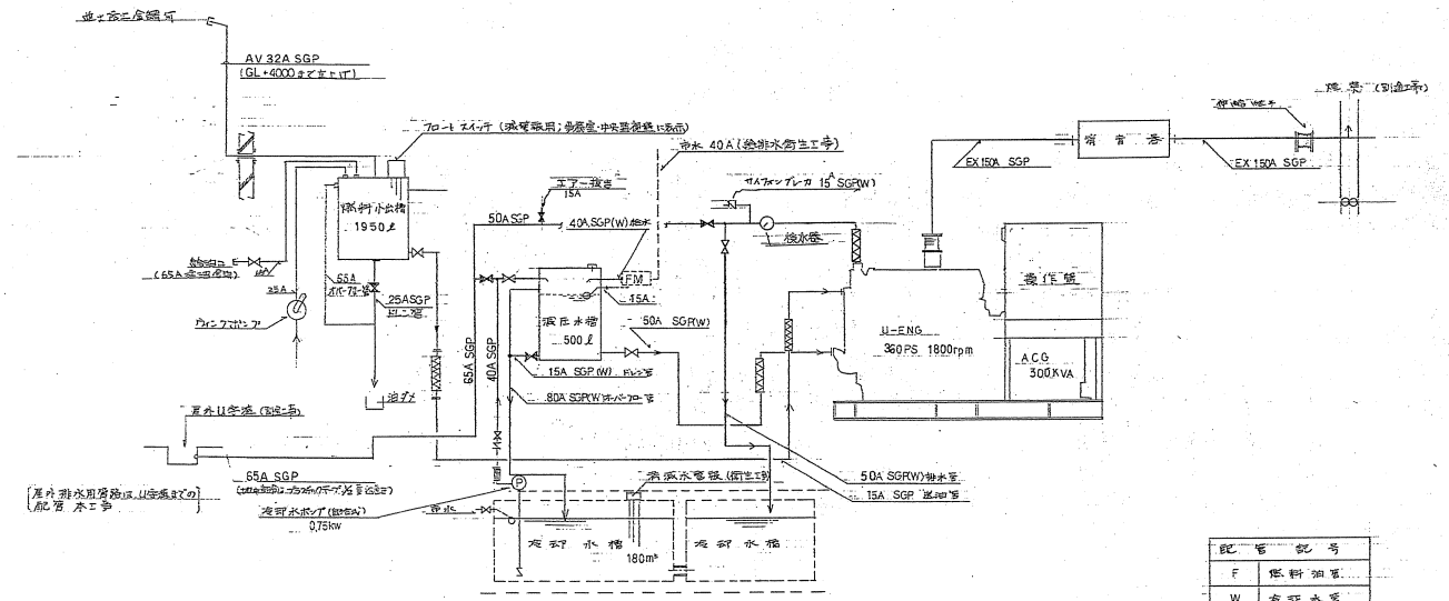
配管系統図 (参考図)
