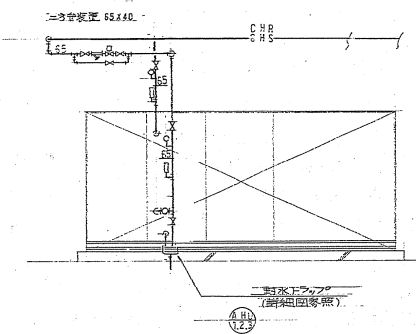
火薬棟 2 階空調機機室 断面図 1/50
