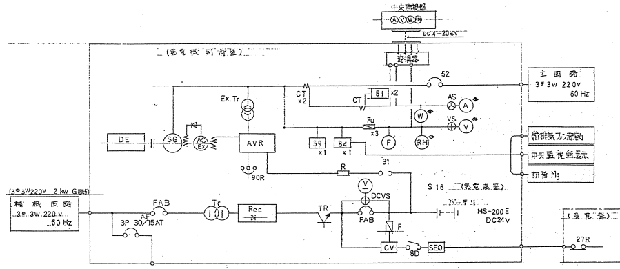
電気配線図 (参考図)
