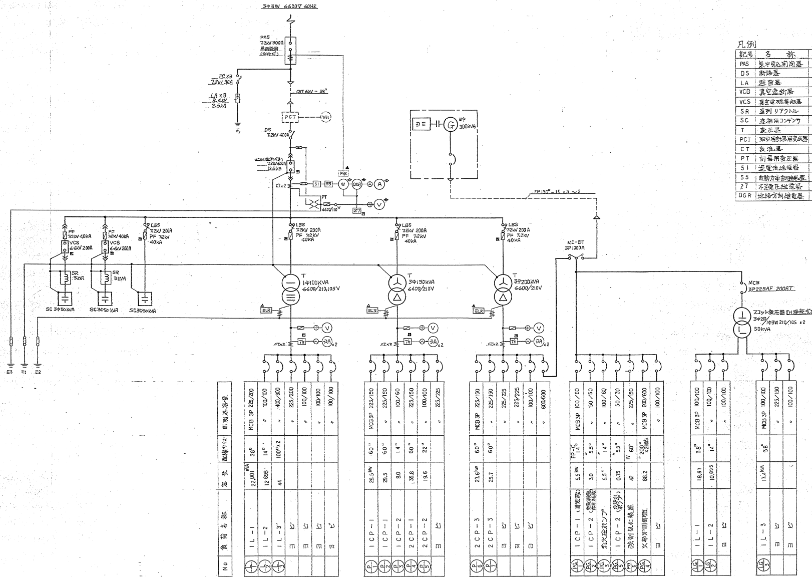
単線回路図
