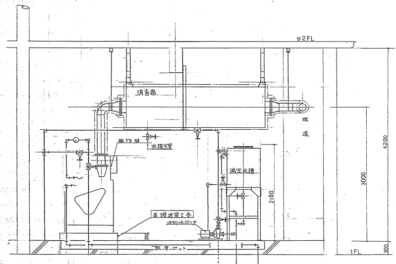
A-A 断面図 1/30 冷却水仕上
