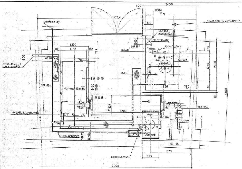
平面配置図 1/30
