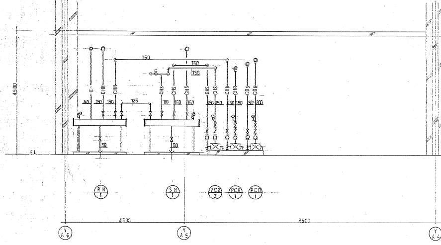
1楼空調機室断面図 1/50
