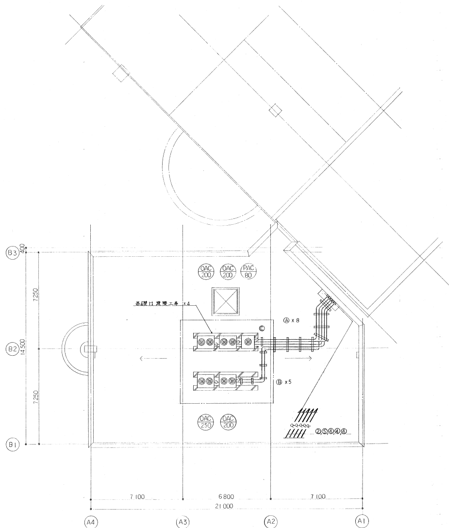
屋上空調配管平面図 S:1/100
