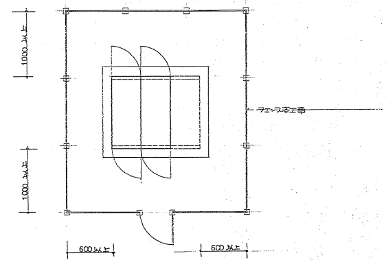
電気室配線図 1/50
