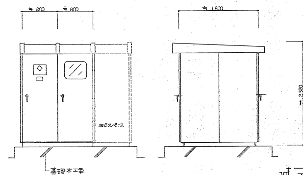
基礎工事
