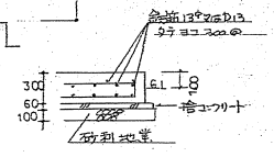
基礎詳細図
