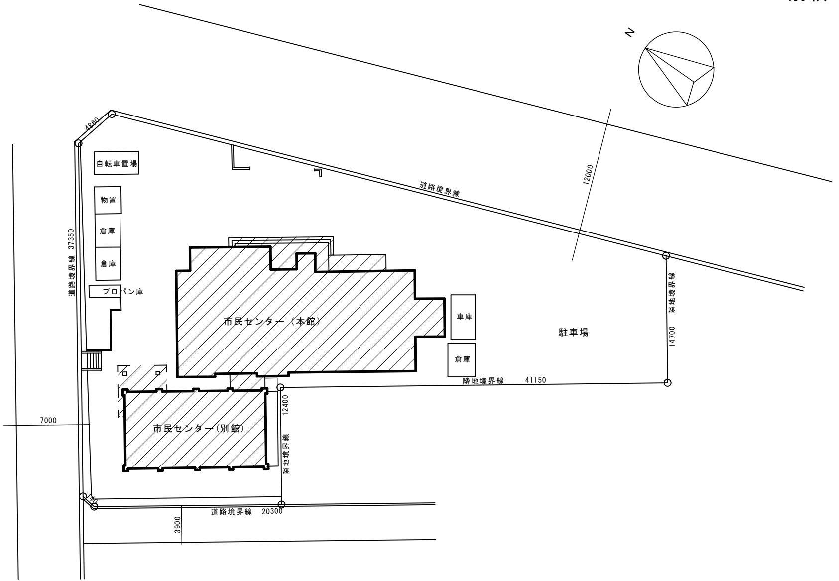
配置図 1 : 200
