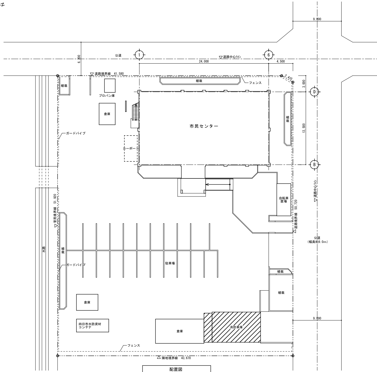
配置図
