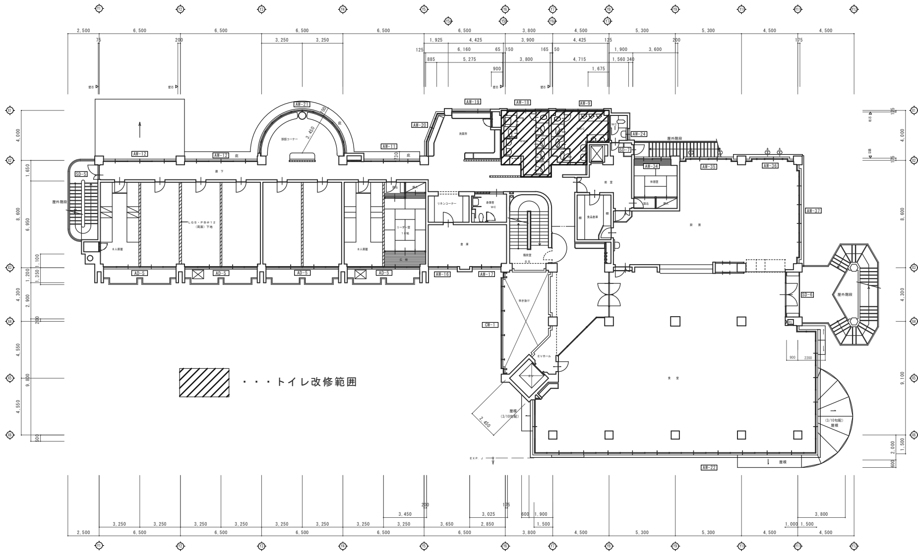
本館2F平面図
