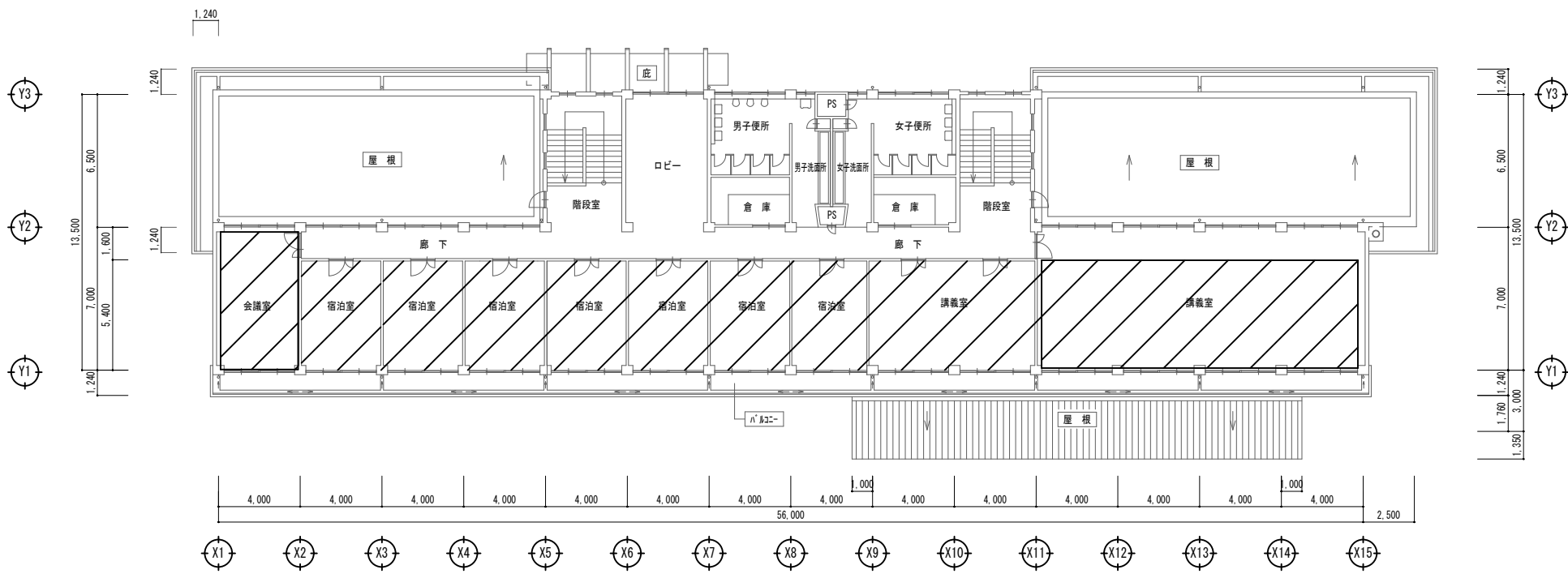
分館2階平面図
