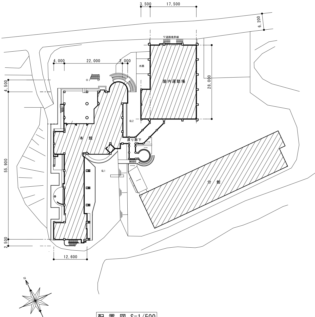
配置図 S=1/500
