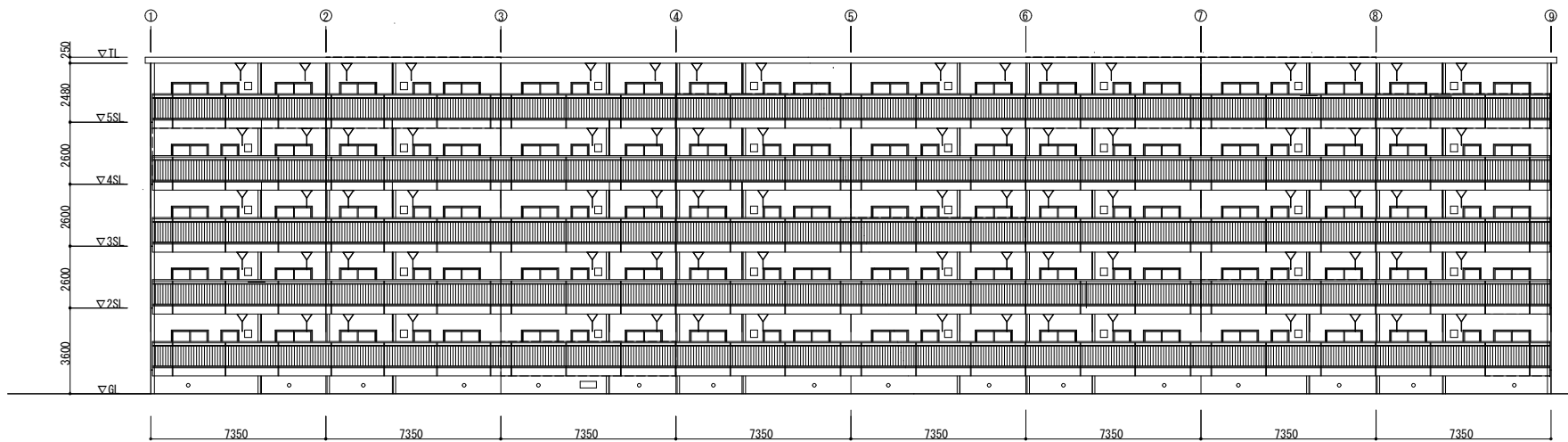
南立面图
