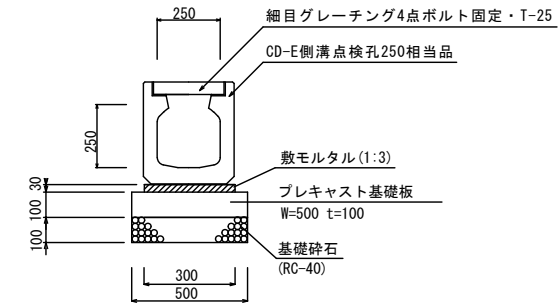
函渠型側溝工(250型) (点検孔) (横断部)
