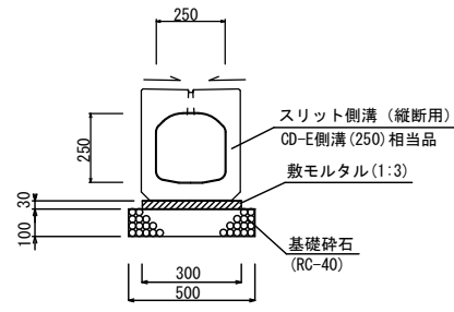
函渠型側溝工(250型) (縦断用)
