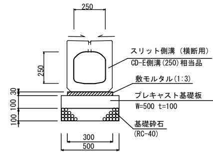
函渠型側溝工(250型) (横断用)
