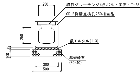
函渠型側溝工(250型) (点検孔) (縦断部)
