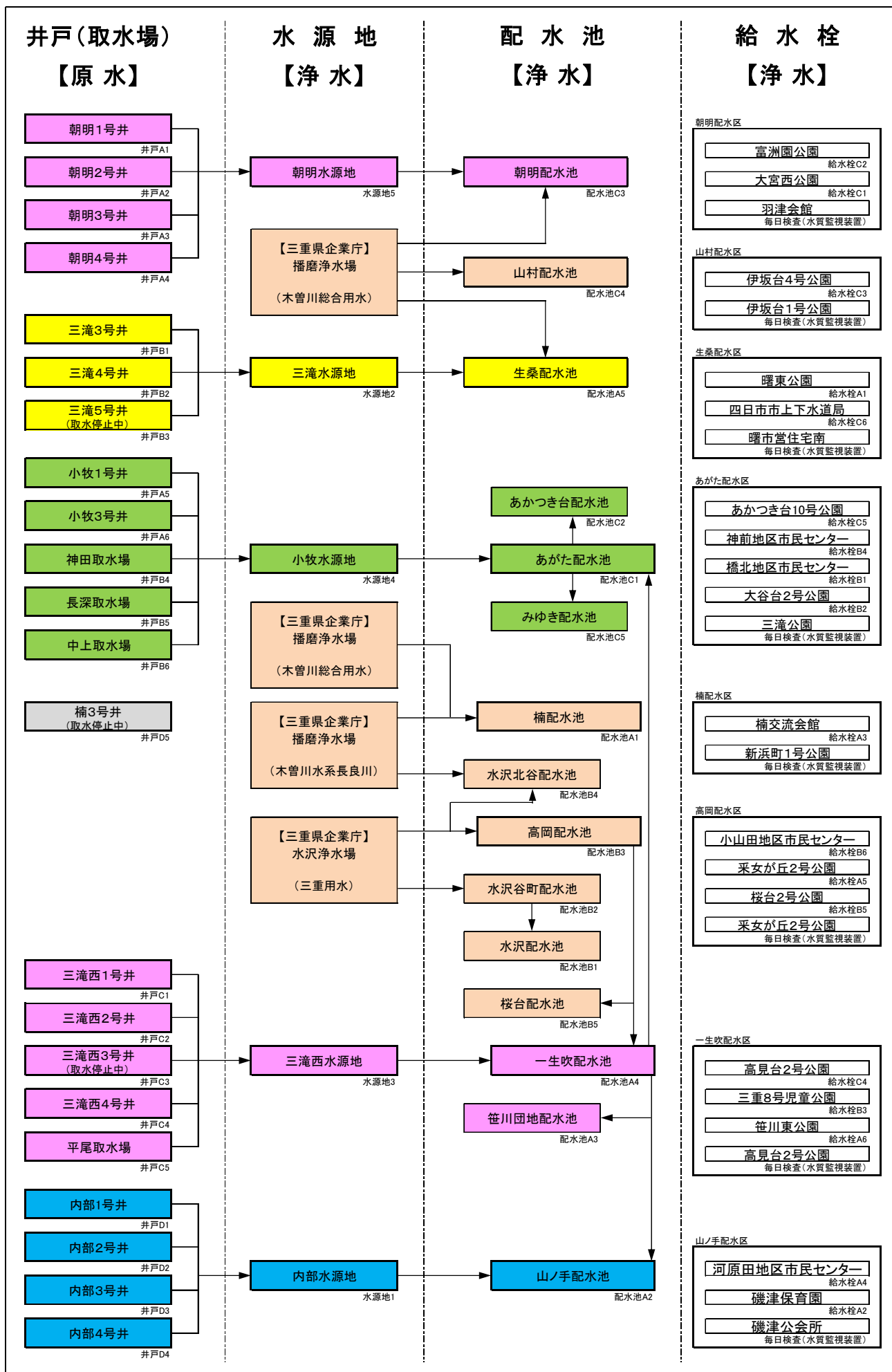
図2 配水系統図
