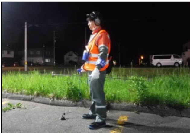
漏水探知の実施状況
