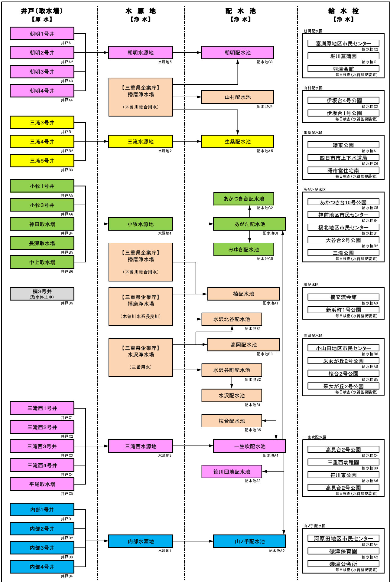
図2 配水系統図
