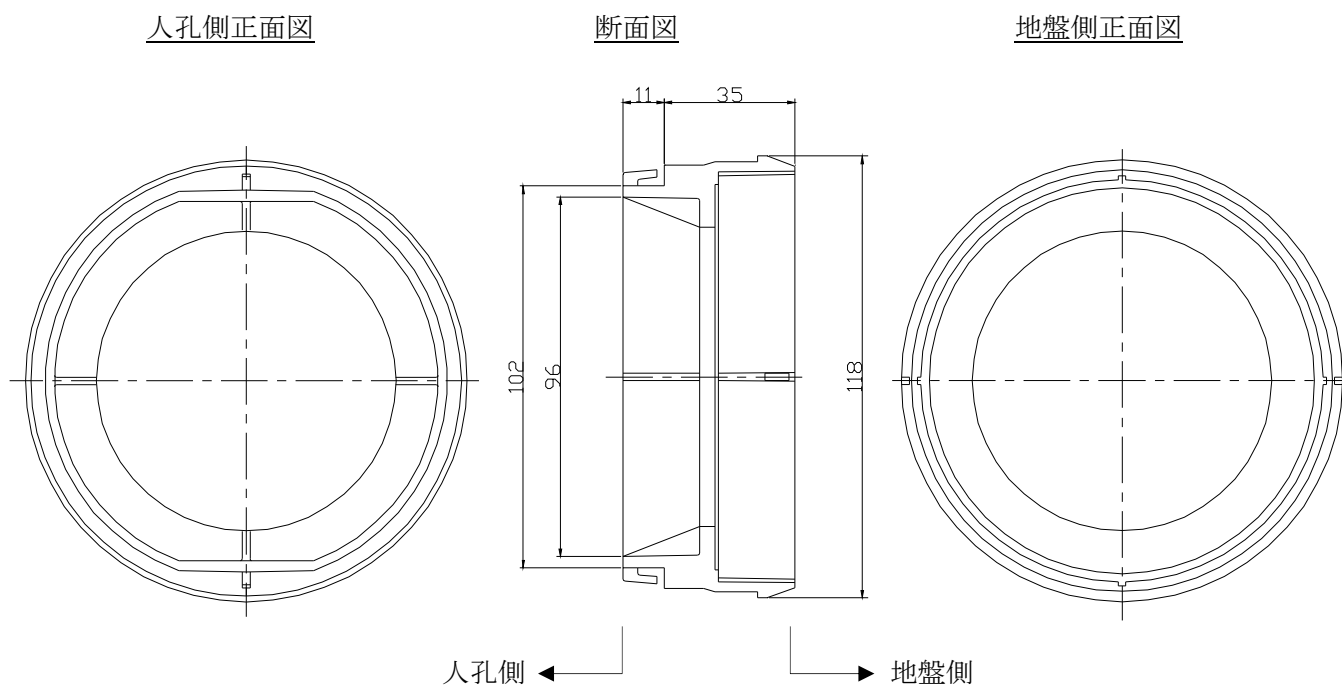
図－２ 延長ソケット構造図
