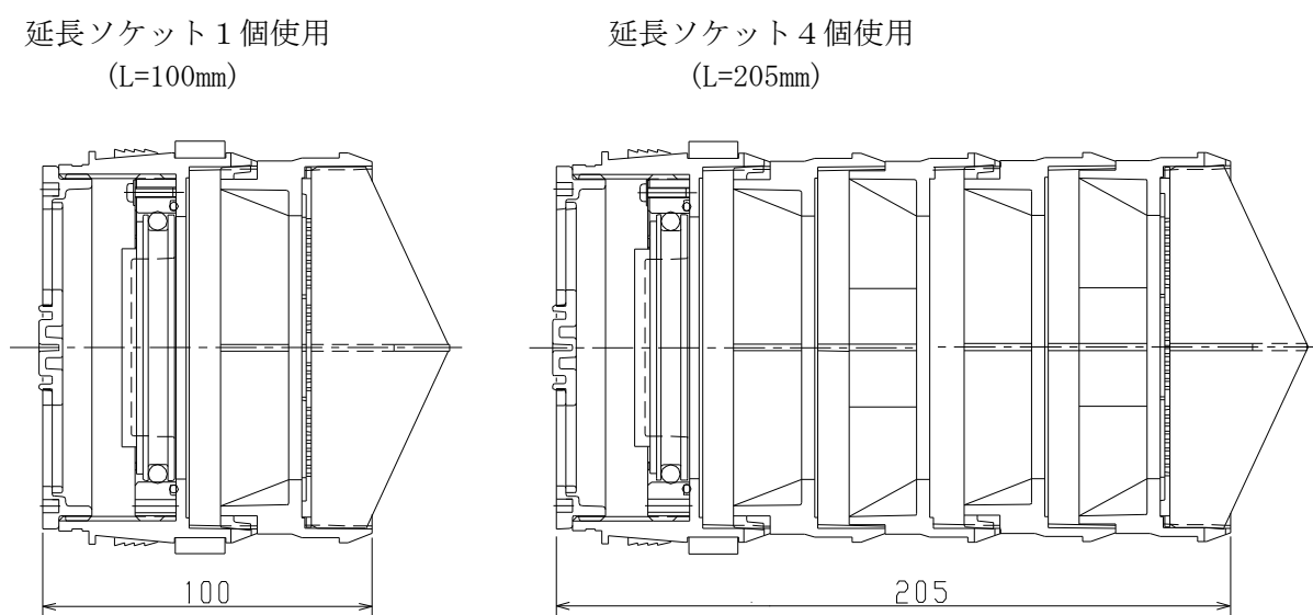
図－３ 参考図（消散弁、延長ソケット接続例）
