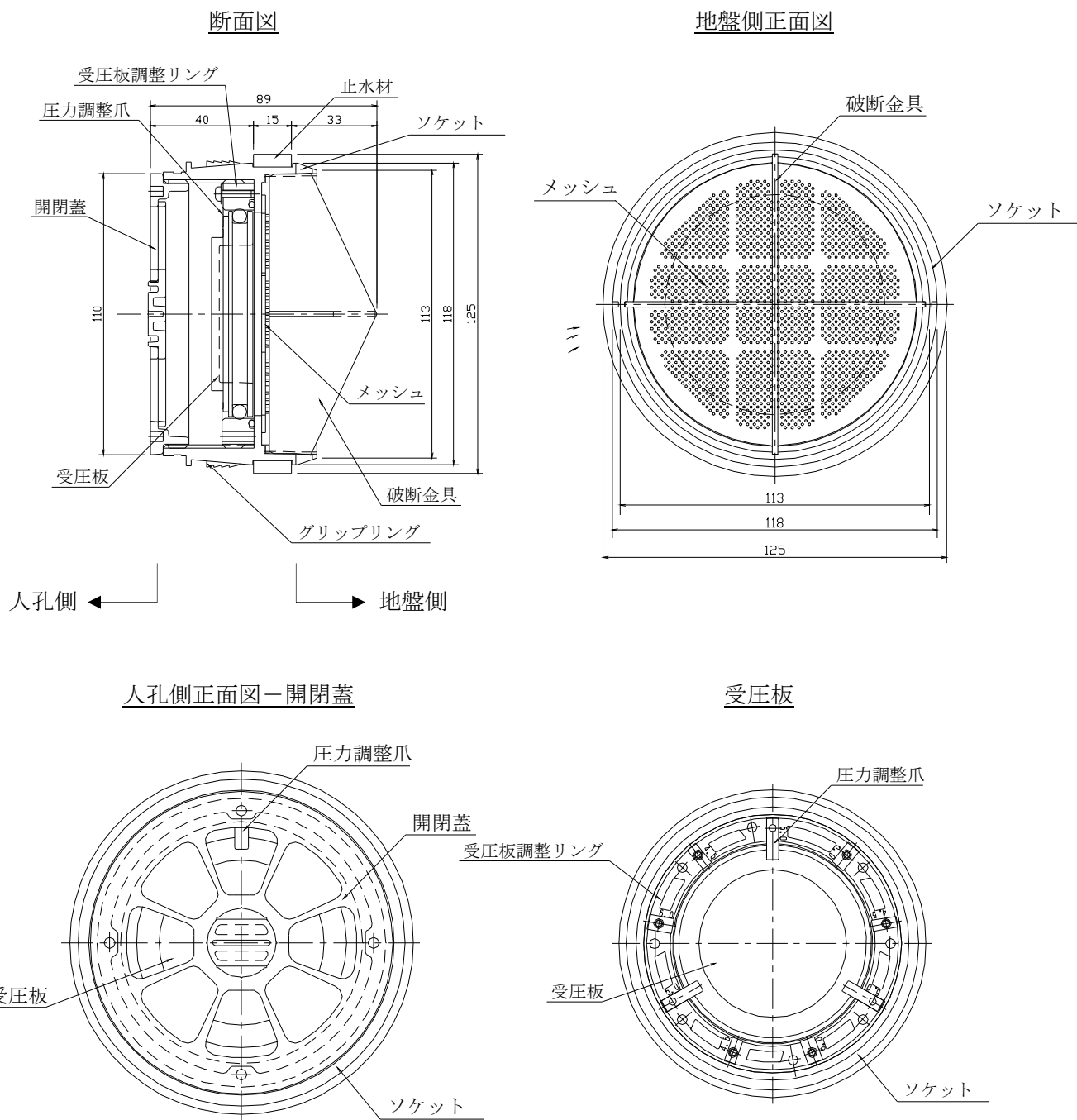
図－１ 消散弁構造図
