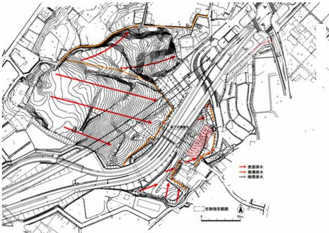
雨水排水施設計画図
