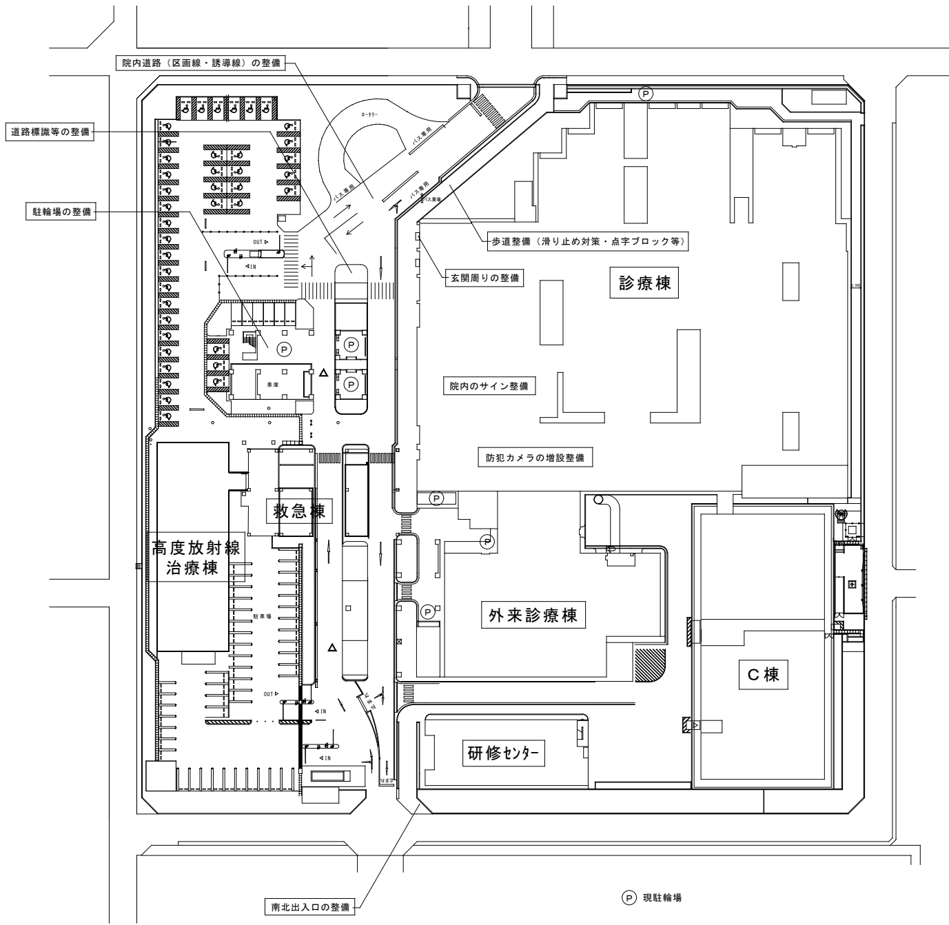
配置図
