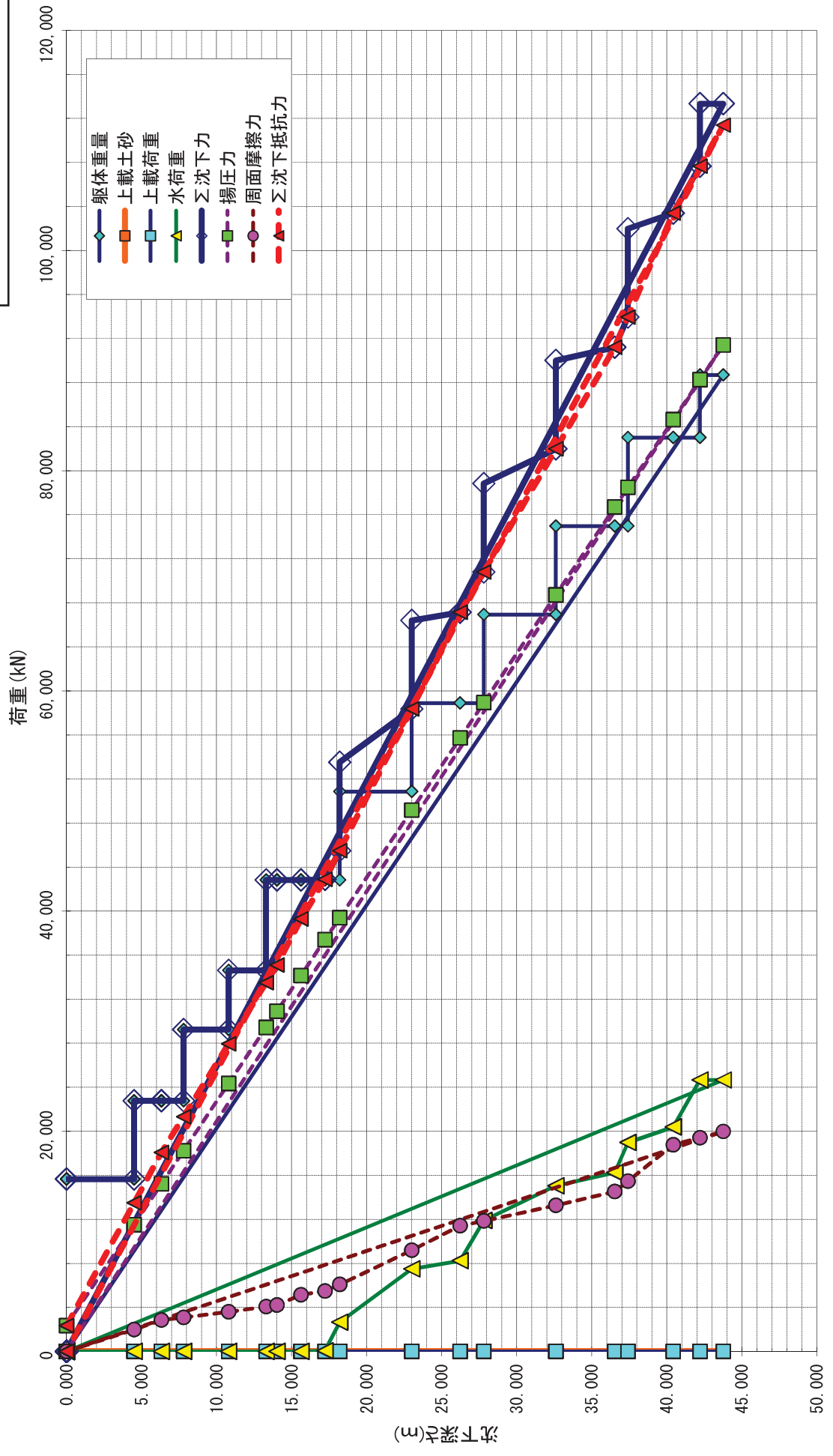
沈下関係図(参考)
