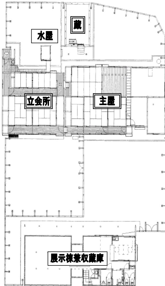
1 階平面図
